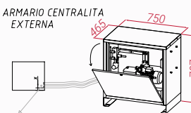
ZONA DE ENTRADA DE CABLES Y TUBOS PROVENIENTES DE LA MAQUINARIA PUNTO DE ENTRADA LINEA ELECTRICA
